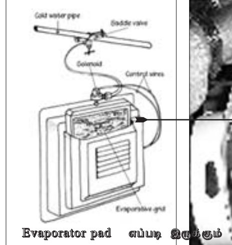
Evaporator pad எப்படி இருக்கும் என்பதை அறிந்து கொள்ளும் படம்
